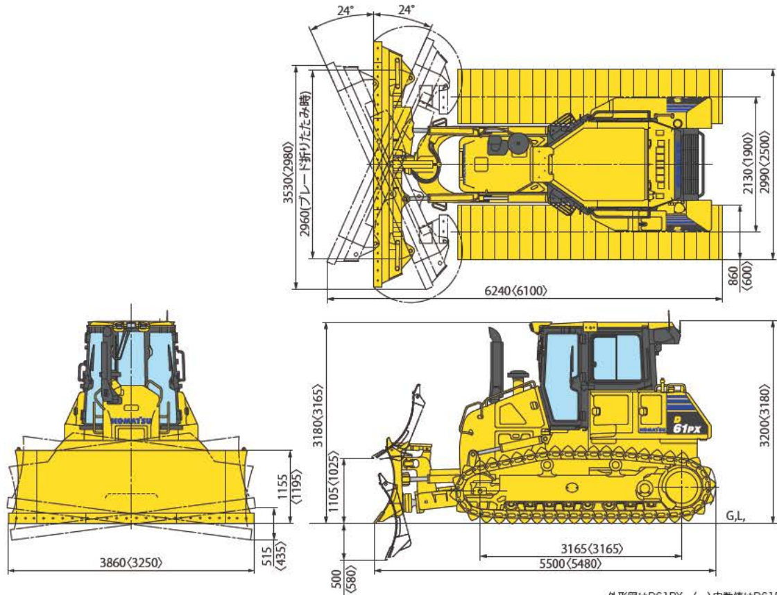
外形図はD61PX、〈 〉内数値はD61EX (単位: mm)
